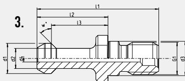
3. ISO 7388-3 Forme JD avec perçage/Form JD with drill through (ancienne norme/previous norm MAS 403 30°/45°)
