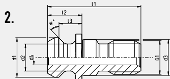
2. ISO 7388-3 Forme UD avec perçage/Form UD with drill through (ancienne norme/previous norm ISO 7388-2 Form B)
