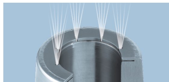
Perçage de conduits d'arrosage optimisé avec sortie du liquide par des fentes. Optimised coolant bores with coolant outlet through slots.
