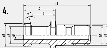
4. JIS B 6339 avec perçage/with drill through
